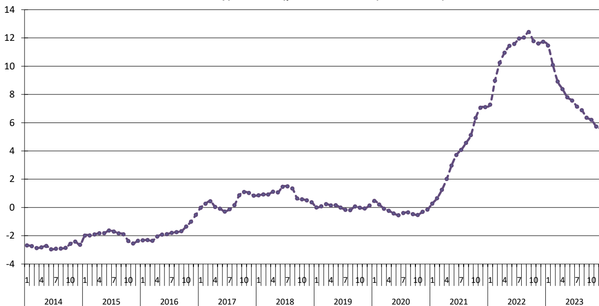
Εξέλιξη ετήσιων μεταβολών (%) Δείκτη Τιμών Υλικών Κατασκευής Νέων Κτηρίων Κατοικιών (2015=100,0)
